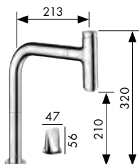
M7119-H200 2-Loch Einhebel-Küchenmischer mit Ausziehauslauf, Schwenkbereich 150° # 73804,-000,-800
