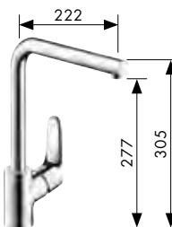
Focus® 280 Einhebel-Küchenmischer mit Schwenkauslauf 110°/150°/360° # 31817,-000
