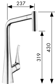
Metris® 320 Einhebel-Küchenmischer mit Ausziehbrause, 2-strahlig, Schwenkauslauf 110°/150° # 14820,-000,-800
