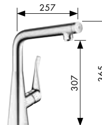
Metris® Select 320 Einhebel-Küchenmischer mit Schwenkauslauf 110°/150°/360° # 14883,-000,-800
