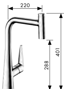
Talis® Select S 300 Einhebel-Küchenmischer mit Ausziehauslauf, Schwenkbereich 150° # 72821,-000,-800
