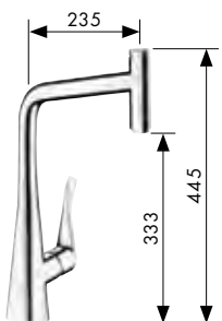
Metris® Select 320 Einhebel-Küchenmischer mit Ausziehauslauf, Schwenkbereich 150° # 14884,-000,-800
