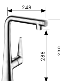
Talis® Select S 300 Einhebel-Küchenmischer mit Schwenkauslauf 110°/150°/360° # 72820,-000,-800
