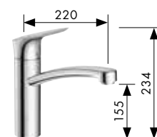
Logis® 160 Einhebel-Küchenmischer mit Schwenkauslauf 360° # 71832,-000 # 71833,-000 für Vorfenstermontage (o. Abb.) # 71834,-000 mit Geräteabsperrventil (o. Abb.) # 71839,-000 CoolStart Eco (o. Abb.)
