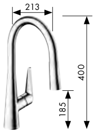
Talis® S 200 Einhebel-Küchenmischer mit Ausziehbrause, 2-strahlig, Schwenkauslauf 110°/150° # 72813,-000,-800
