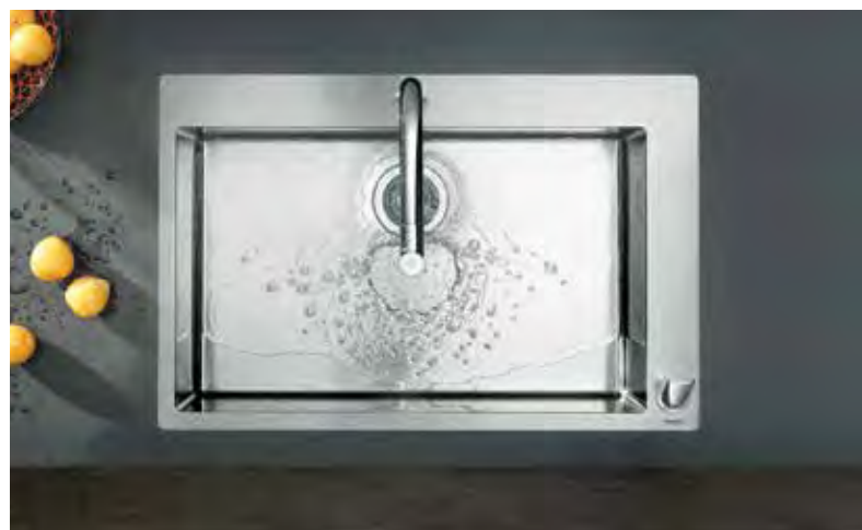
Einbauspüle S711-F660 Die komfortable Spüle mit extrabreitem Becken. Maße: Spüle 760 x 500 mm, Becken 660 x 400 mm, Tiefe 190 mm, für Einbauschrank 800 mm.
