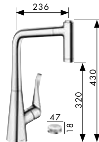
M7120-H320 2-Loch Einhebel-Küchenmischer mit Ausziehrause und 2 Strahlarten # 73806,-000,-800
