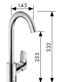
Logis® 260 Einhebel-Küchenmischer mit Schwenkauslauf 110°/150°/360° # 71835,-000
