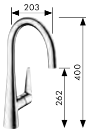
Talis® S 260 Einhebel-Küchenmischer mit Schwenkauslauf 110°/150°/360° # 72810,-000,-800 # 72812,-000 für offene Warmwasserbereiter
